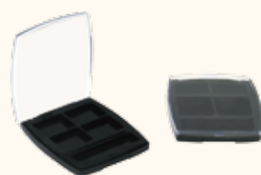
Item No: LB-118A L/W/H: 74.1*66.10*15.10mm Size of well: 25.00*18.30*4.00mm*4 /50.99*10.79*4.00mm
